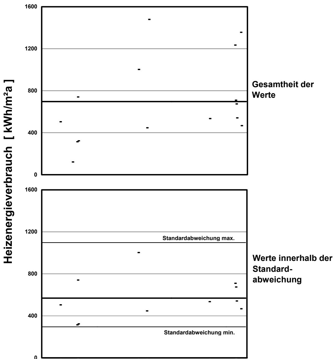
Bild 13: Gegenüberstellung des Heizenergieverbrauchs der Außenanlagen an Universitäten als Gesamtheit der Werte (Bild oben) und als Werte innerhalb der Standardabweichung (Bild unten) mit den jeweiligen Mittelwerten.
