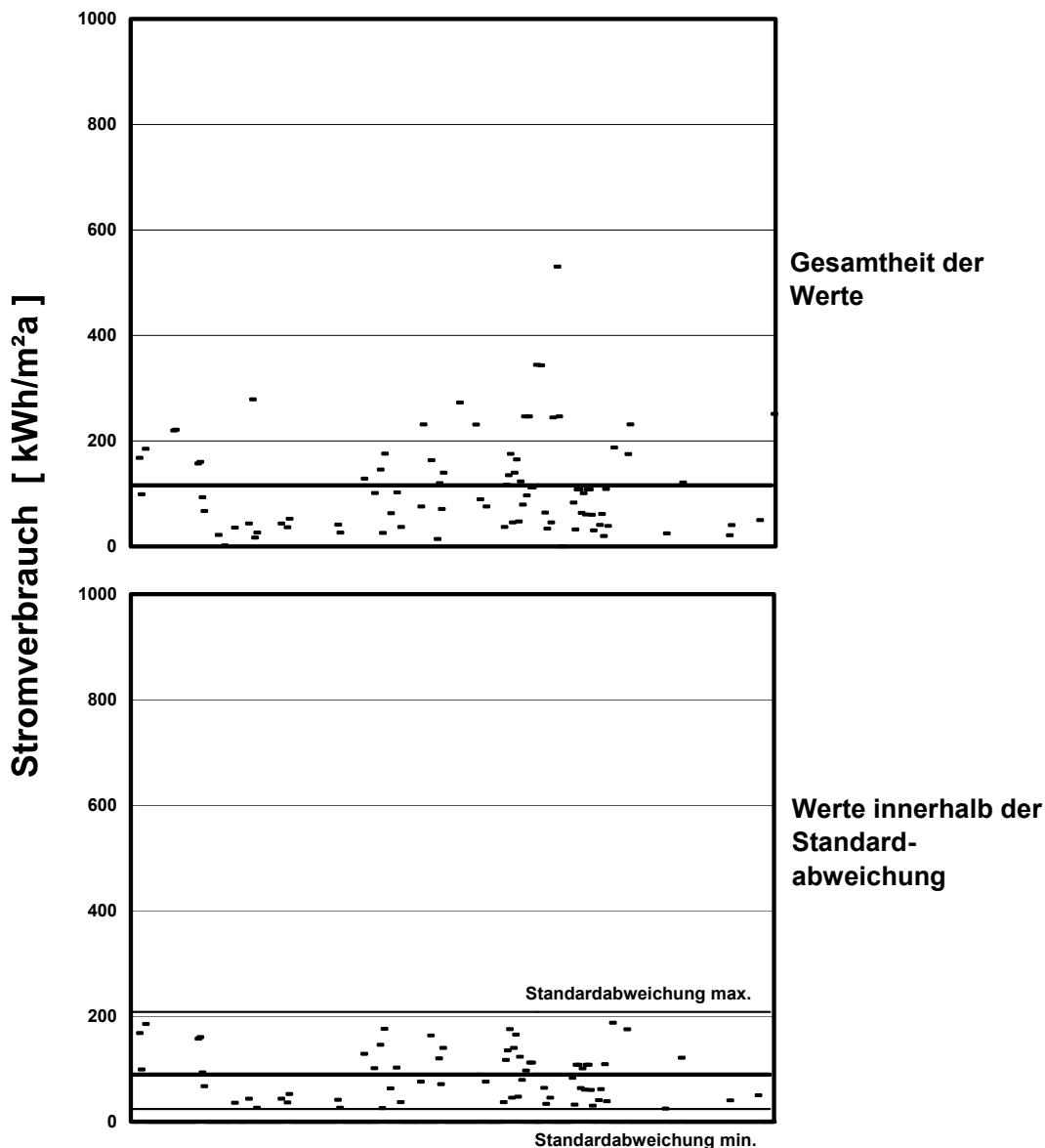
Bild 22: Gegenüberstellung des Stromverbrauchs von ingenieurwissenschaftlichen und von sonstigen naturwissenschaftlichen Institutsgebäuden an Universitäten als Gesamtheit der Werte (Bild oben) und als Werte innerhalb der Standardabweichung (Bild unten) mit den jeweiligen Mittelwerten.
