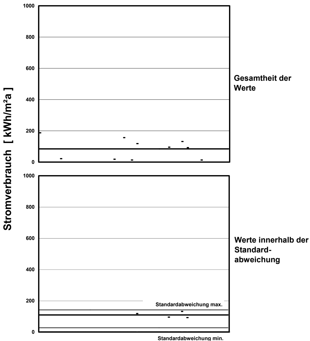
Bild 23: Gegenüberstellung des Stromverbrauchs der Hörsäle an Universitäten als Gesamtheit der Werte (Bild oben) und als Werte innerhalb der Standardabweichung (Bild unten) mit den jeweiligen Mittelwerten.
