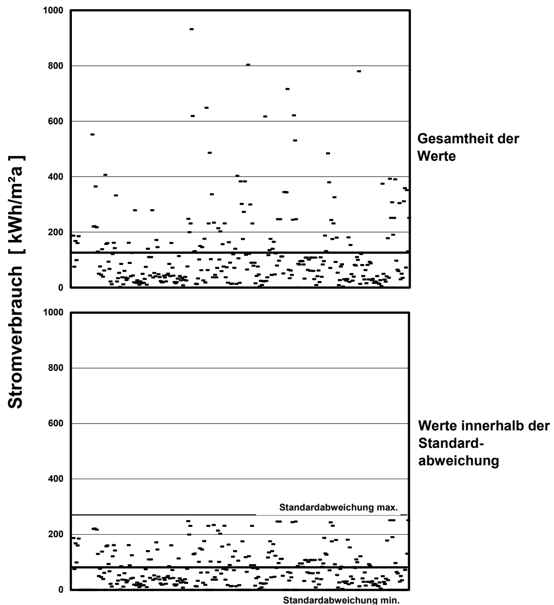
Bild 19: Gegenüberstellung des Stromverbrauchs von Universitätsgebäuden als Gesamtheit der Werte (Bild oben) und als Werte innerhalb der Standardabweichung (Bild unten) mit den jeweiligen Mittelwerten.
