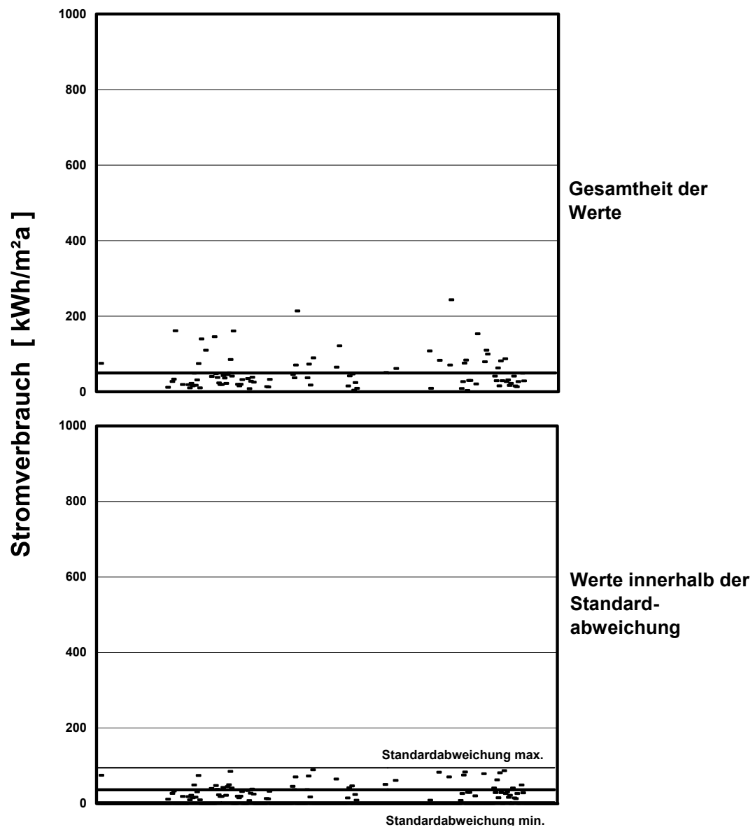
Bild 20: Gegenüberstellung des Stromverbrauchs von geisteswissenschaftlichen Institutsgebäuden an Universitäten als Gesamtheit der Werte (Bild oben) und als Werte innerhalb der Standardabweichung (Bild unten) mit den jeweiligen Mittelwerten.
