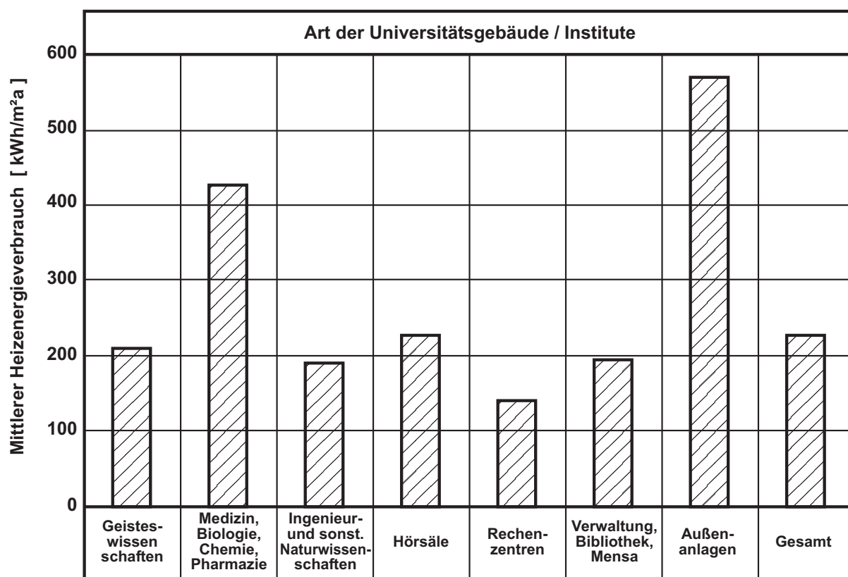
Bild 28: Mittelwerte des Heizenergieverbrauchs der Daten innerhalb der Standardabweichung für die verschiedenen Universitätsgebäudearten.
