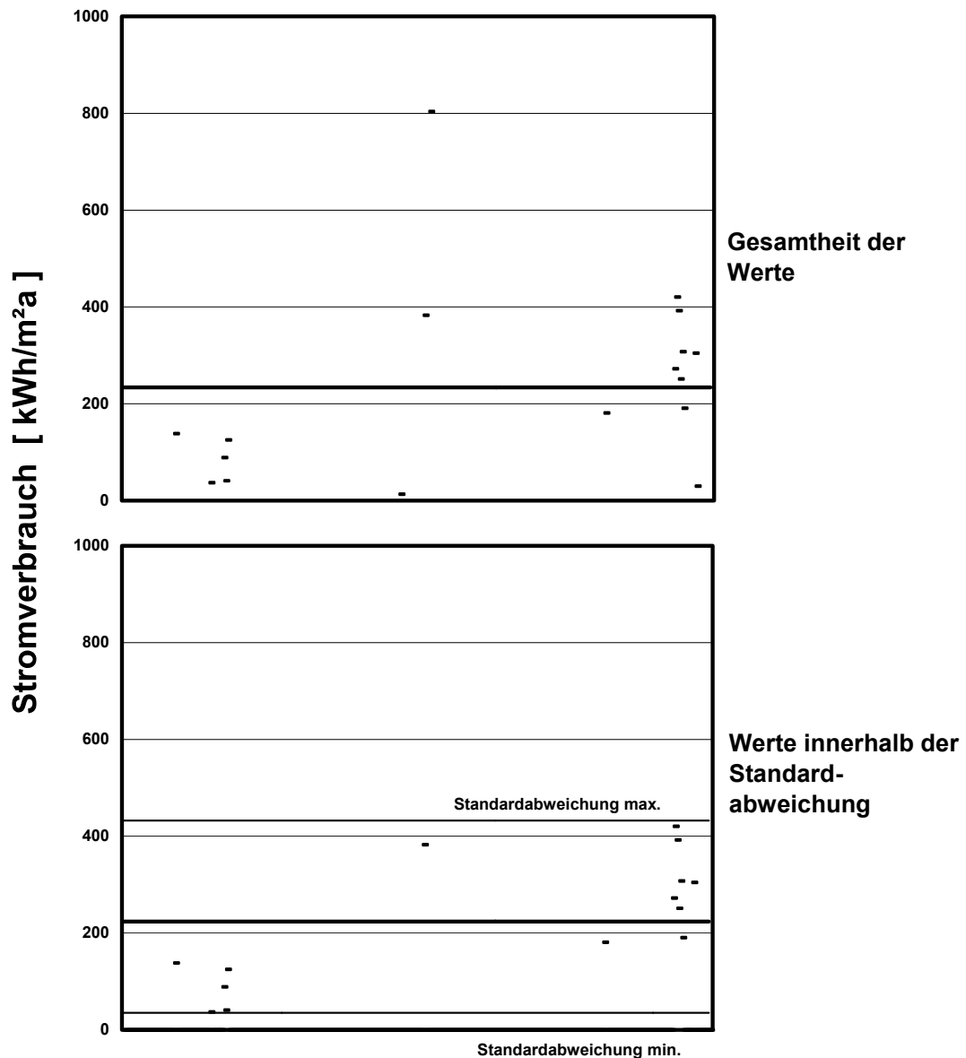
Bild 26: Gegenüberstellung des Stromverbrauchs der Außenanlagen an Universitäten als Gesamtheit der Werte (Bild oben) und als Werte innerhalb der Standardabweichung (Bild unten) mit den jeweiligen Mittelwerten.
