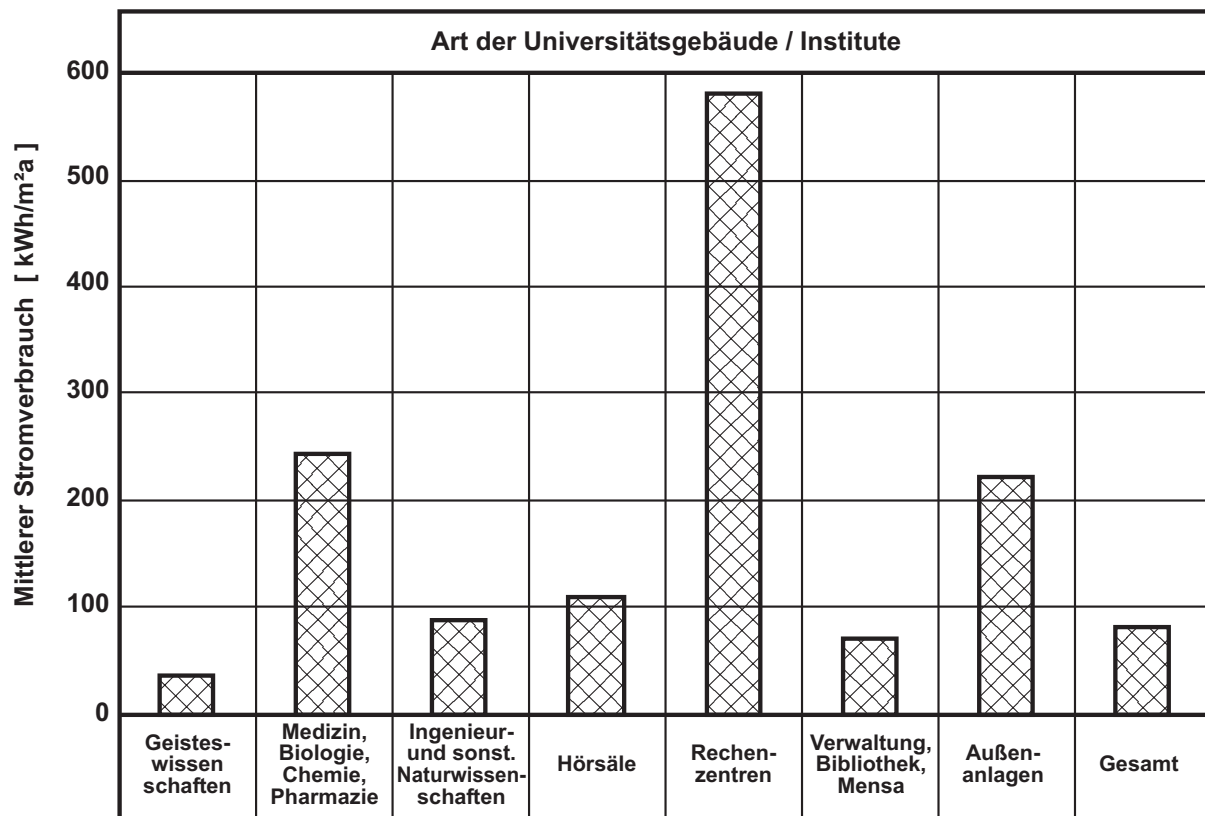
Bild 30: Mittelwerte des Stromverbrauchs der Daten innerhalb der Standardabweichung für die verschiedenen Universitätsgebäudearten.
