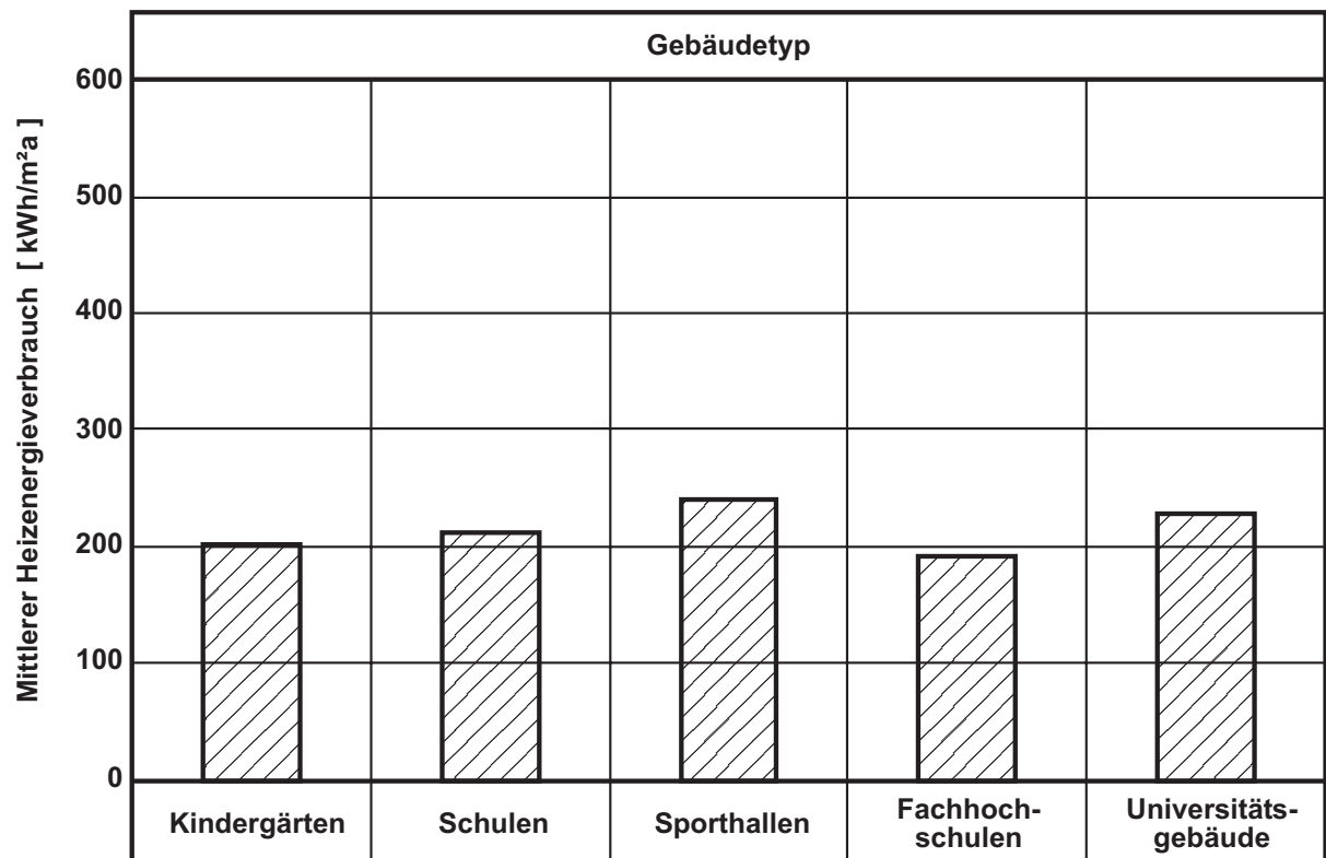
Bild 27: Mittelwerte des Heizenergieverbrauchs der Daten innerhalb der Standardabweichung für die verschiedenen Bildungsgebäudetypen.
