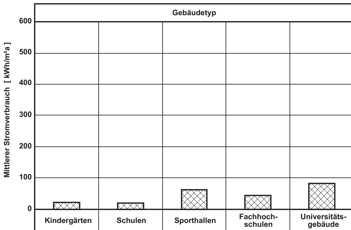
Bild 29: Mittelwerte des Stromverbrauchs der Daten innerhalb der Standardabweichung für die verschiedenen Bildungsgebäudetypen.
