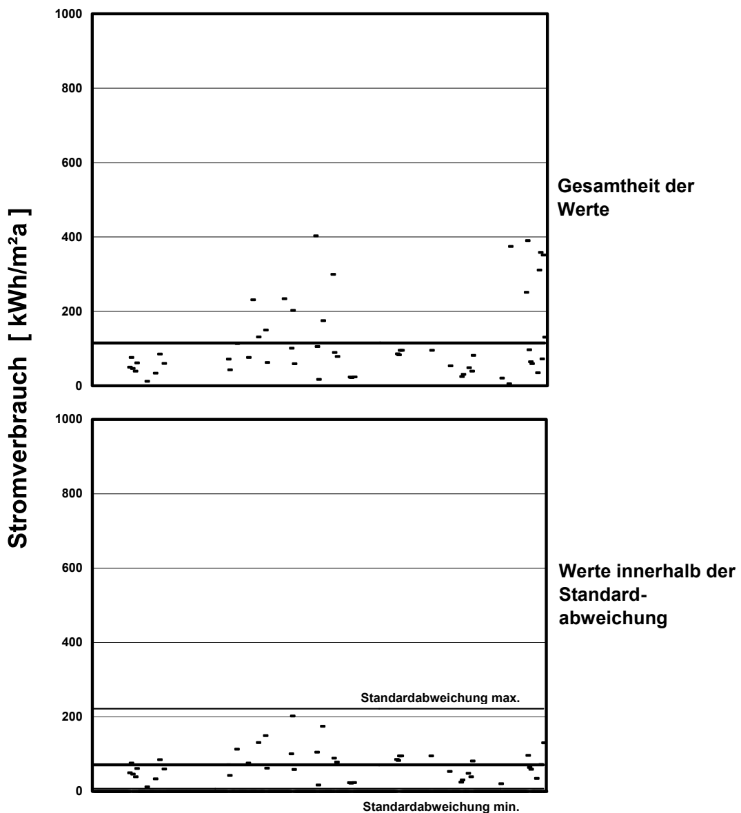
Bild 25: Gegenüberstellung des Stromverbrauchs der Verwaltungen, Bibliotheken und Mensen an Universitäten als Gesamtheit der Werte (Bild oben) und als Werte innerhalb der Standardabweichung (Bild unten) mit den jeweiligen Mittelwerten.
